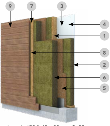
1. Trestenderverk (C24) 48 x 98 mm 2. 98 mm ROCKWOOL Flexi A-plate 34 3. Dampspærre 4. 2 lag 12,5 mm gipsplate type A 5. 18 mm OSB 6. 100 mm ROCKWOOL Redair plate 7. ROCKWOOL Redair Flex LVL og FP 8. ROCKWOOL Redair Flex W skruer 9. Valgfri utvendig kledning
