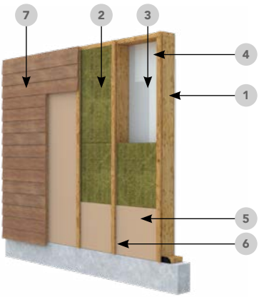
1. Trestenderverk (C24) 48 x 198 mm 2. 198 mm ROCKWOOL Flexi A-plate 34 3. Dampspærre 4. 12,5 mm gipsplate type A 5. 9,5 mm gipsplate type EH2 6. 23x48 mm trelekter 7. 19 mm trekledning
