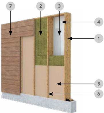
1. Trestenderverk (C24) 36 x 198 mm 2. 198 mm ROCKWOOL Flexi A-plate 34 3. Dampspærre 4. 12,5 mm gipsplate type A 5. 9,5 mm gipsplate type EH2 6. 23 x 48 mm trelekter 7. 19 mm trekledning
