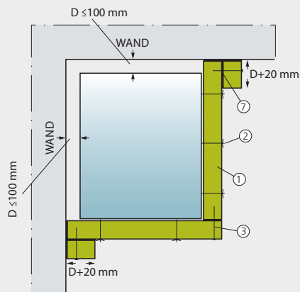
Dwarsdoorsnede verticaal luchtkanaal met 2-zijdige bekleding
