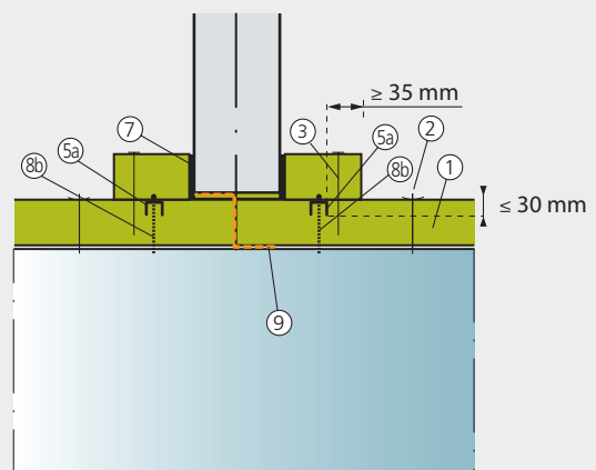
Detail muurdoorvoering, massieve wand
