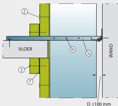
Langsdoorsnede verticaal luchtkanaal met 2-zijdige bekleding
