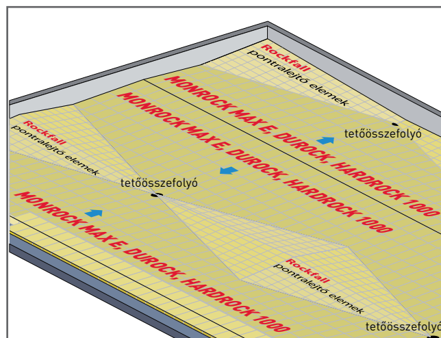
A tervezett legfelső inhomogén hőszigetelő lemezek, például MONROCK MAX E, DUROCK, HARDROCK 1000 elhelyezése után a ROCKFALL pontralejtő elemek elhelyezése fektetési terv alapján. A pontralejtő elemek segítségével megoldható az ellenlejtés az összefolyó és az attikafal között.
