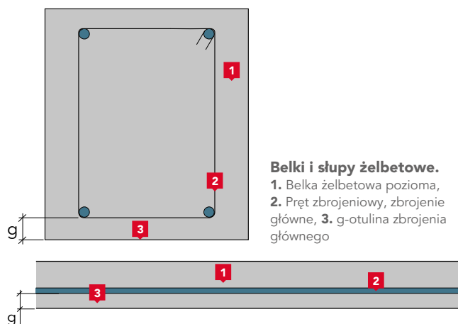
Przekrój przez strop żelbetowy. 1. Strop żelbetowy, 2. Pręt zbrojeniowy, zbrojenie główne, 3. g-otulina zbrojenia głównego
